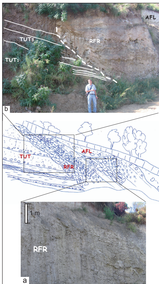
Fig. 60 - a) detriti stratificati e cementati del sistema di Raffo Rosso (RFR). b) contatto erosivo dei depositi dei sistemi RFR e AFL con le sottostanti Tufiti di Tusa (membro marnoso e membro arenaceo). Le intercalazioni cm-dm di marne micacee laminate ( TUT_1 ) passano verso l'alto alle arenarie verdastre ( TUT_3 ). Il limite tra le due unità litostatigrafiche è graduale come risulta dalla diminuzione verso l'alto delle intercalazioni marnose. Il Capo, versante nord di Poggio Maria.
