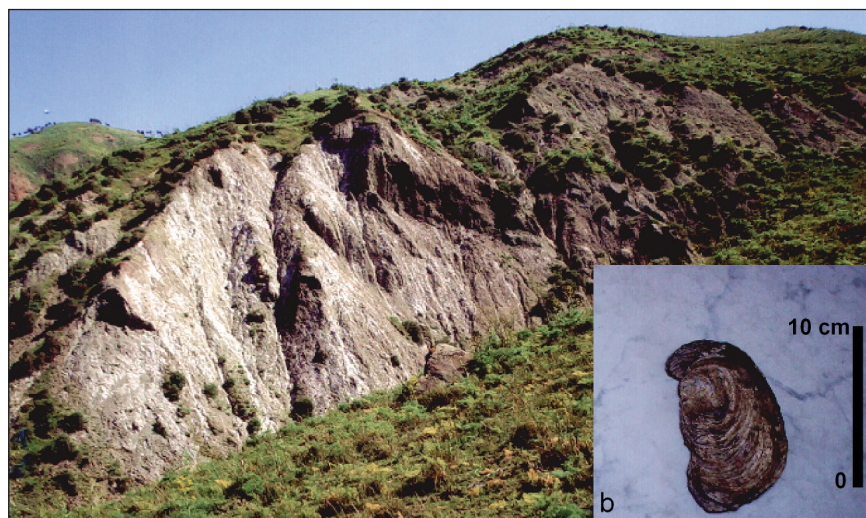
Fig. 13 - Affioramento delle marne ad Exogira nelle argille varicolori inferiori ("Cenomaniano in facies africana"); b) particolare di Exogira sp. Contrada Cinci, Caltavuturo.
