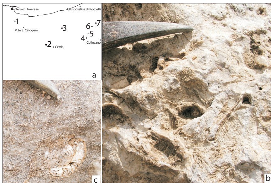
Fig. 14 - a) Ubicazione dei corpi di breccie a caprinidi (AVF) intercalate nelle AVF: 1, Torrente Tre pietre; 2, Torre del Principe; 3, Rocca del Drago; 4, Serra Canalona; 5, Rocca Sciacchi di Gatto; 6, Rocca di Uoni; 7, Cozzo S. Agata. b) Breccie carbonatiche con caprinidi e briozoi intercalate nei livelli cenomaniani delle AVF. c) Dettaglio di rudiste. Torre del Principe (dintorni di Sciara).
