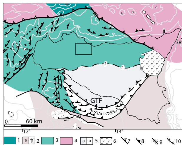
Fig. 7 - Carta strutturale della Sicilia e delle aree marine contermini (modificata da CATALANO et alii , 1996). 1) unità tettoniche kabilo sarde; 2) crosta continentale africana(a), carbonati clastici del Miocene (b); 3) unità Siculo-Maghrebidi; 4) unità Kabilo-Calabridi; 5) Falda di Gela (a), avanfossa plio-pleistocenica (b); 6) Vulcaniti; 7) faglie inverse; 8) fronti di sovrascorrimento; 9) Faglie trascorrenti; 10) Faglie dirette; GTF: Gela Thrust Front.
