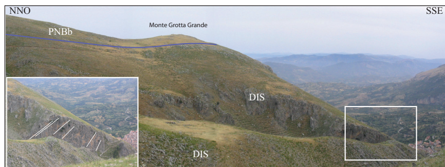
Fig. 40 - Panoramica del contatto stratigrafico tra i calcari di Piano Battaglia (PNBb) e le sottostanti Dolomie di Isnello (DIS).
