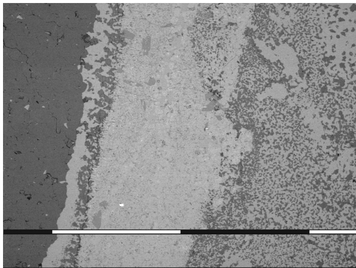
Fig. 75 - Breccia del Pissalat (BPA). Microfotografia SEM. Da sinistra verso destra: clasto di dolomite, banda di calcite e silicati (centro), zona a calcite (chiara) e dolomite (scura); (scala di riferimento = 1 mm).
