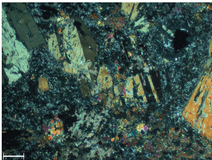
Fig. 65 - Filone lamprofirico basaltico (fu). Microfotografia a polarizzatori incrociati. Struttura porfirica con fenocristalli idiomorfi di orneblenda in pasta di fondo minuta (scala di riferimento 350 \mu\text{m} ).
