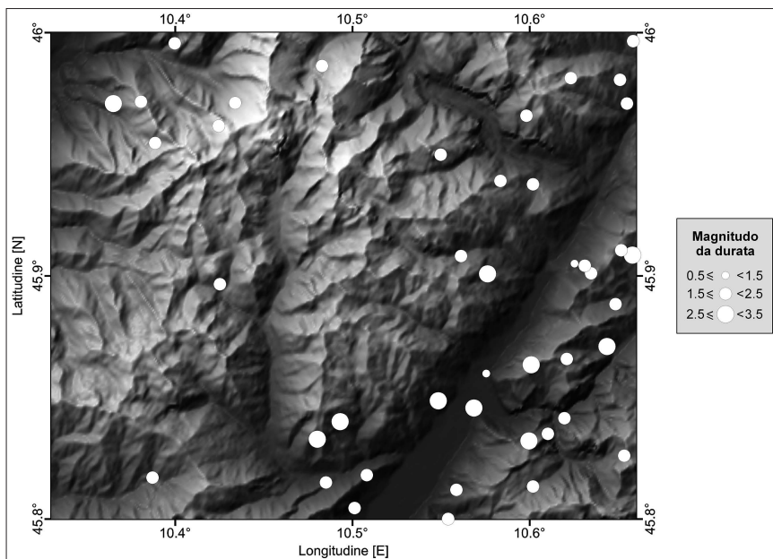
Fig. 94 - Sismicità strumentale all'interno dell'area di studio, nel periodo 1991-2008. Localizzazioni dal bollettino sismico della rete sismometrica della Provincia Autonoma di Trento.
