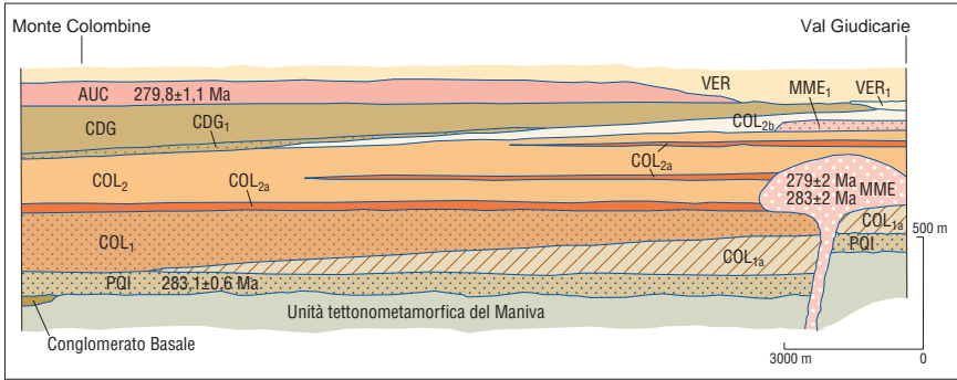
Fig. 54 - Schema stratigrafico del Gruppo delle Tre Valli Bresciane.
