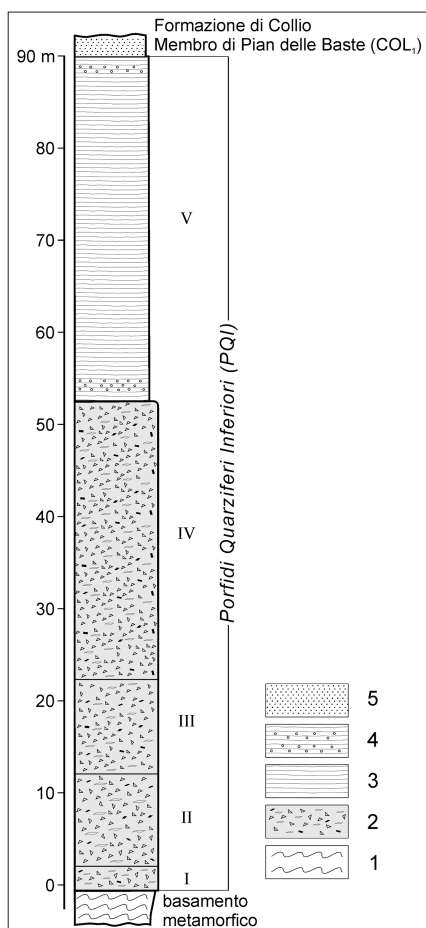
Fig. 30 - Colonna stratigrafica della formazione dei porfidi quarziferi inferiori (PQI). Affioramento di Cascinello dei Zocchi lungo la SS 345 Maniva - Croce Domini. 1 - basamento metamorfico. 2 - ignimbrite. 3 - tufo. 4 - tufo con lapilli di accrezionamento. 5 - arenaria. Modificato da BERTOZZI (1996).
