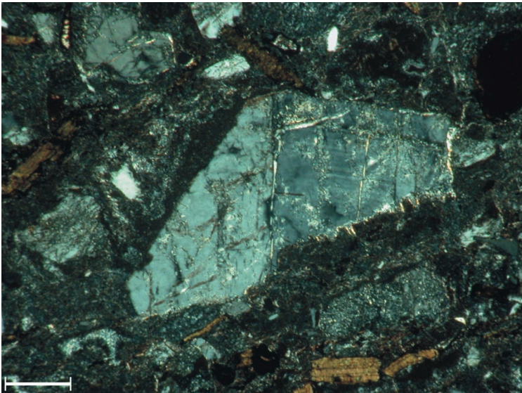
Fig. 52 - Vulcanite di Auccia - Litozona superiore. Particolare di cristallo di K-feldspato (sanidino). Microfoto a polarizzatori incrociati (scala di riferimento 250 \mu\text{m} ).
