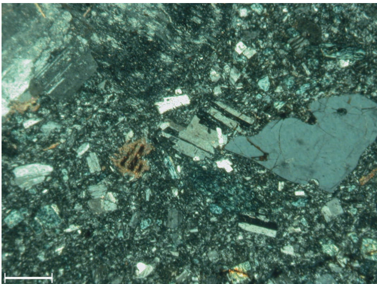
Fig. 41 - Formazione di Monte Macaone. Particolare con plagioclasto, pirosseno, biotite e quarzo. Microfoto a polarizzatori incrociati (scala di riferimento 125 \mu\text{m} ).
