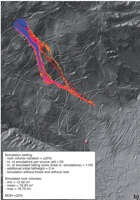
Fig. 97 - a) Rappresentazione del rilievo tramite GPS della traiettoria principale (riferita al masso di maggiore volume) della frana complessa (scivolamento rotazionale evoluto in crolli), che ha interessato la zona di Faserno, nei pressi di Storo, nel dicembre 2010. b) simulazione del crollo elaborato tramite il programma "Rockyfor 3D", in cui sono rappresentate le possibili traiettorie e la frequenza dei passaggi dei massi. In blu è rappresentata la massima frequenza di passaggio.
