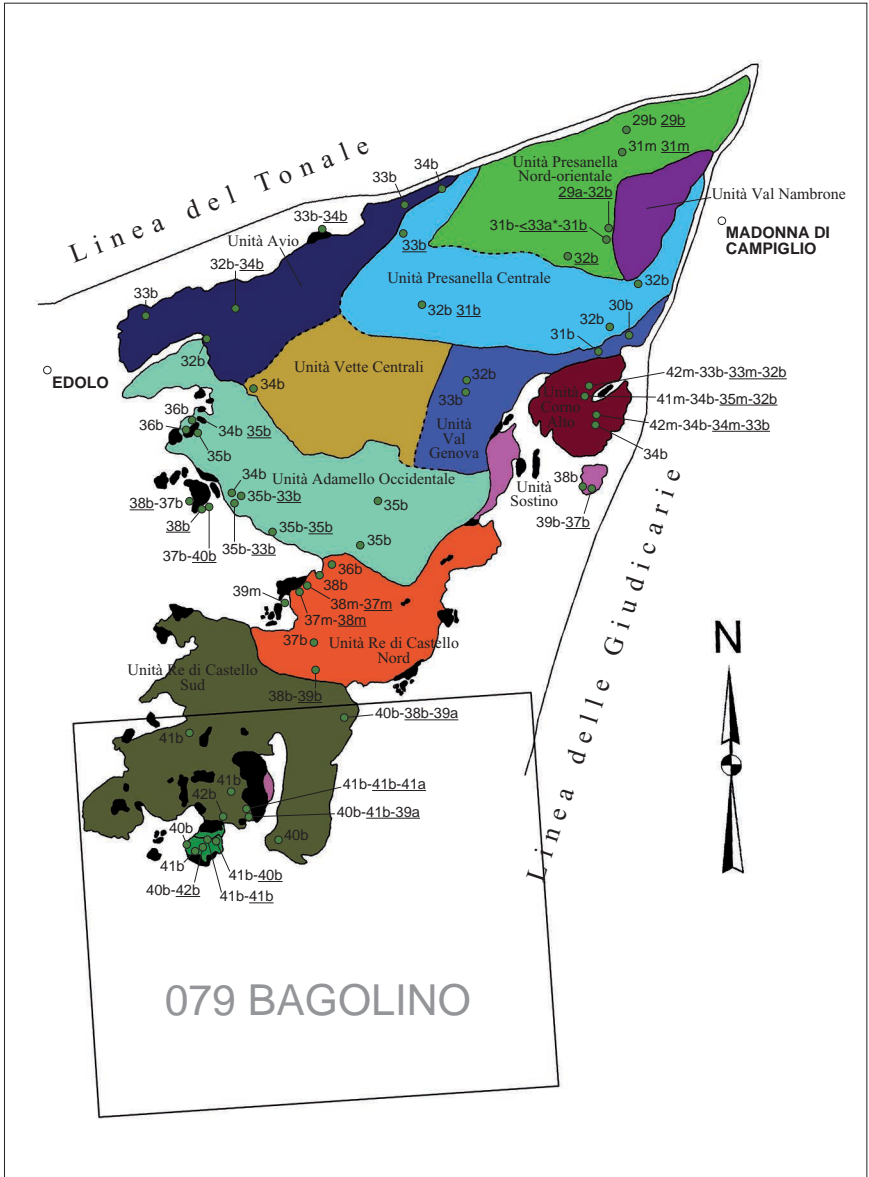
Fig. 6 - Schema geologico del batolite dell'Adamello e dati cronologici (modificato da DEL MORO et alii, 1985a). Abbreviazioni: (m) e (b) = età sulla muscovite e biotite con metodo Rb/Sr; (m) e (b) = età sulla muscovite e biotite con metodo K/Ar; (a) = età sull'orneblenda con metodo K/Ar; (a*) = età sull'orneblenda con metodo ^{40}\text{Ar}/^{39}\text{Ar} . In nero le masse femiche. La cornice indica la posizione del Foglio 079-Bagolino.
