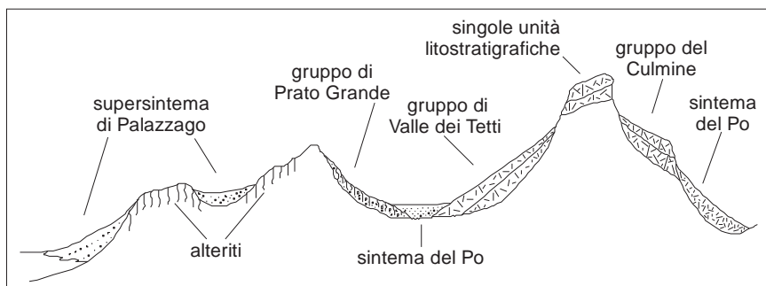
Fig. 2 - Unità non distinte in base al bacino di appartenenza: schema dei rapporti stratigrafici dei depositi di versante al raccordo versanti-pianura e in media valle.
