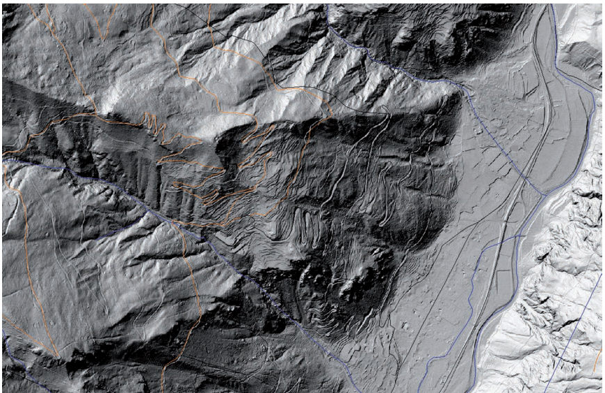
Fig. 104 - Estratto del modello digitale del terreno tramite il rilievo LIDAR, in cui si osserva la morfologia della frana che caratterizza il versante in corrispondenza dell'abitato di Brione.
