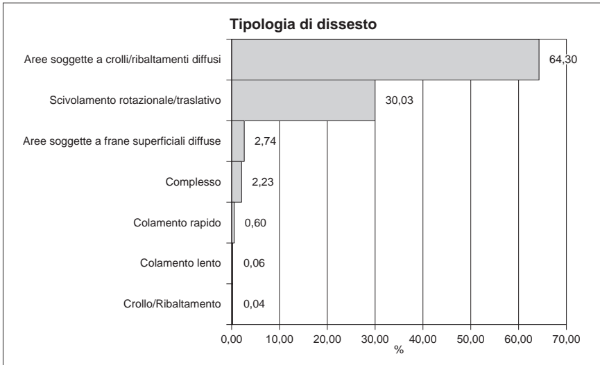
Fig. 95 - Distribuzione percentuale delle diverse tipologie di dissesto nel settore lombardo del Foglio.
