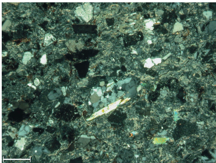
Fig. 50 - Vulcanite di Auccia - Litozona superiore. Ignimbrite con xenoliti di basamento. Microfoto a polarizzatori incrociati (scala di riferimento 675 \mu m).
