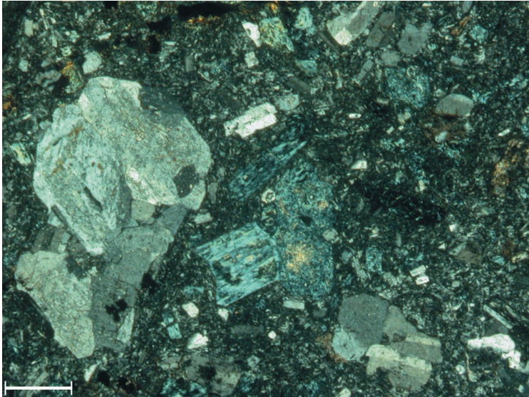
Fig. 40 - Formazione di Monte Macaone. Lava andesitica. Particolare di pirosseni e plagioclasti. Microfoto a polarizzatori incrociati (scala di riferimento 125 \mu\text{m} ).
