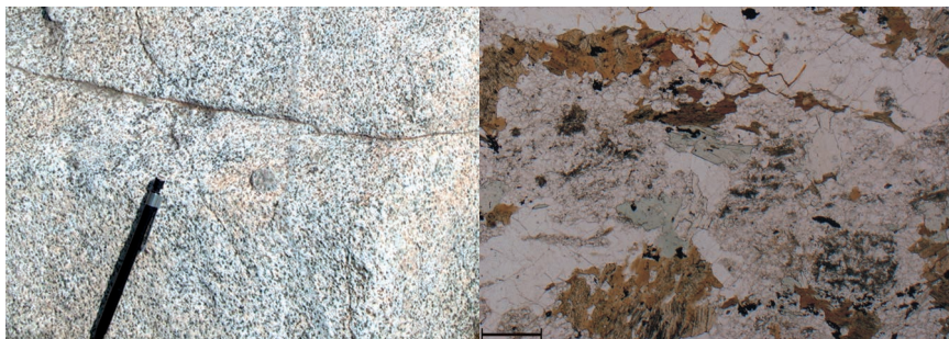
Fig. 28 - Ortogneiss affiorante a Pian delle Baste (a sinistra, foto S. Racchetti) e microfoto a polarizzatori paralleli (a destra) (scala di riferimento 1 mm).
