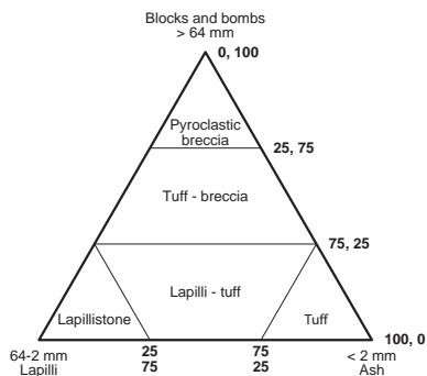
Fig. 31 - Diagramma classificativo dei frammenti piroclastici (da FISHER & SCHMINCKE, 1984).
