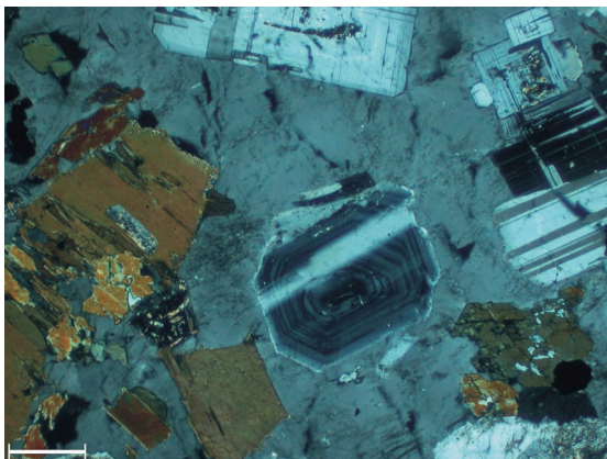
Fig. 72 - Granodiorite della leucotonalite-granodiorite del Lago Boazzo (LBO). Microfotografia a polarizzatori incrociati. Struttura eterogranulare ipidiomorfa con plagioclasti labradoritico-oligoclastici, biotite, orneblenda, K-feldspato e quarzo (scala di riferimento 350 \mu m).
