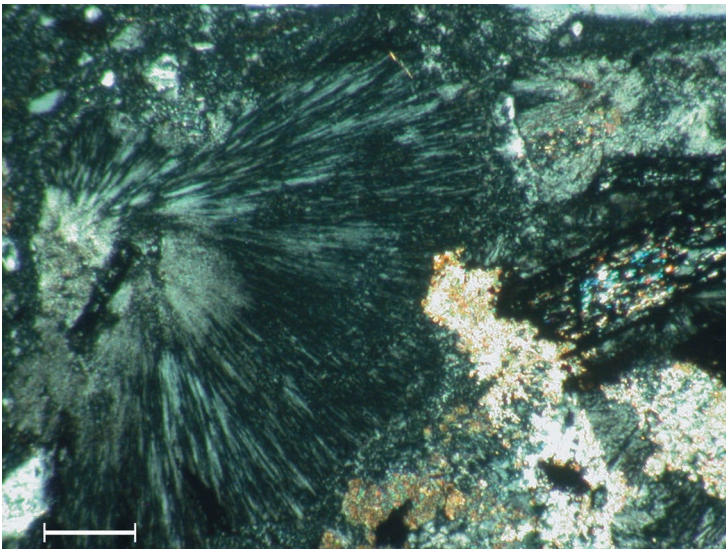
Fig. 49 - Vulcanite di Auccia - Litozona inferiore e intermedia (CASSINIS 1966c). Particolare del fondo ricristallizzato fibroso concentrico raggiato con devetrificazione della componente vetrosa. Microfoto a polarizzatori incrociati (scala di riferimento 675 \mu\text{m} ).
