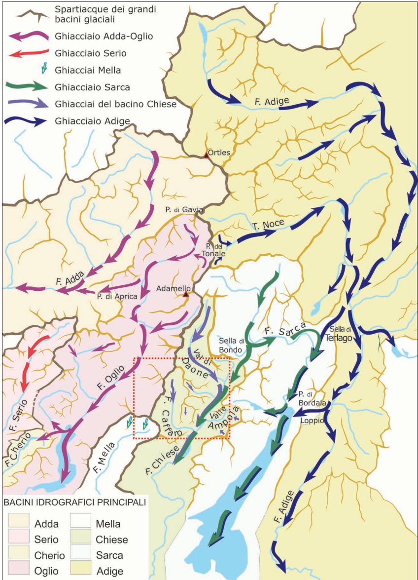
Fig. 18 - Inquadramento del Foglio 079-Bagolino (rettangolo rosso) rispetto ai grandi ghiacciai dell'Oglio e dell'Adige durante l'LGM: i depositi glaciali a oriente dello spartiacque principale afferiscono al supersintema dell'Adige, qui proposto per la prima volta. Dati ricavati dai Fogli 057-Malonno, 058-Monte Adamello, 059-Tione di Trento, 060-Trento, 078-Breno, 080-Riva del Garda, 099-Iseo, 041-Ponte di Legno (SERVIZIO GEOLOGICO D'ITALIA 2012a, 2008, 2005a, 2010, 2012b, 2005b, 2011, 2012c).
