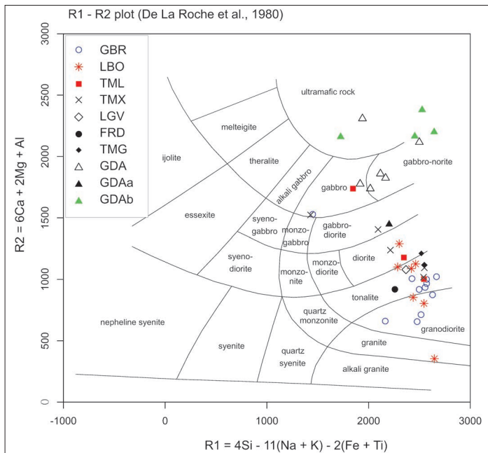
Fig. 73 - Classificazione delle rocce intrusive del plutone Re di Castello nel Foglio 079-Bagolino.
