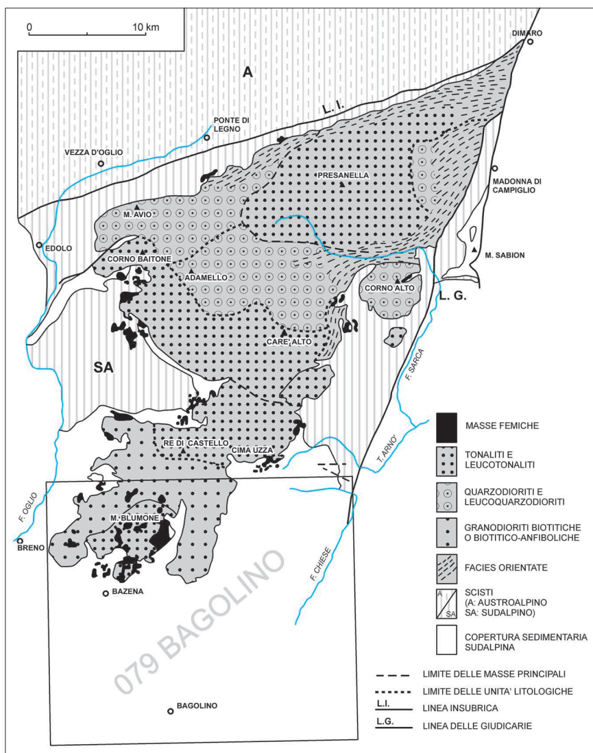
Fig. 5 - Le principali unità intrusive dell'Adamello (modificata da BIANCHI et alii, 1970). La cornice indica l'area del Foglio 079-Bagolino.
