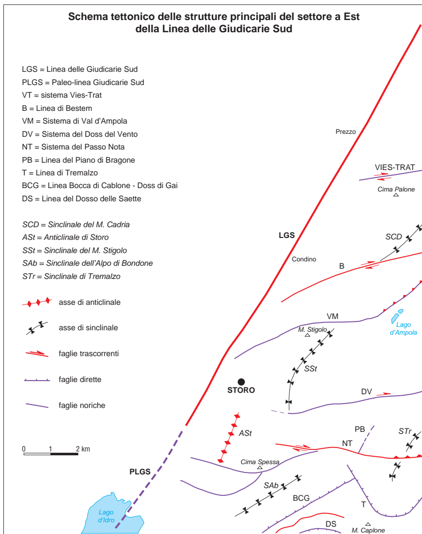
Fig. 93 - Schema tettonico delle strutture principali a E delle Giudicarie.
