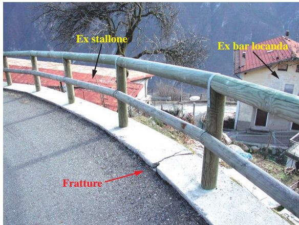
Fig. 102 - Panoramica ripresa da monte della porzione di versante compresa tra l'ex stallone e l'ex bar locanda, con in evidenza le fratture riconducibili al fenomeno franoso in atto.
