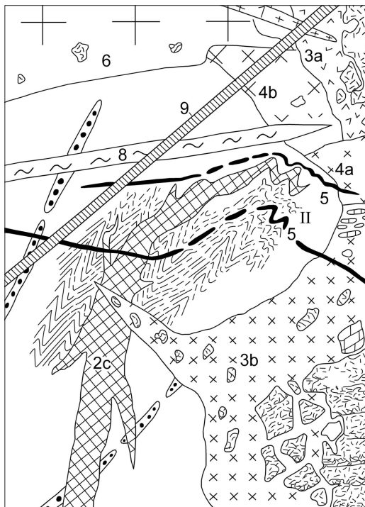
Fig. 10 - Schema dei rapporti mesoscopici tra le deformazioni (I: pieghe pre-intrusione; II: pieghe disarmoniche e boudinage sin-intrusione) e le principali intrusioni al margine meridionale del Massiccio Re di Castello.
