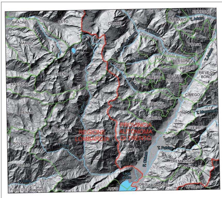
Fig. 1 - Inquadramento geografico-amministrativo del Foglio 079-Bagolino alla scala 1:50.000.
