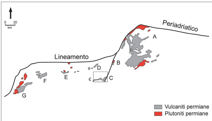
Fig. 4 - Distribuzione delle vulcaniti e delle plutoniti permiane nelle Alpi Meridionali. La cornice racchiude l'area del Foglio 079-Bagolino. A- Trentino Alto Adige e zona di Monte Luco (Gruppo Vulcanico Atesino, GA). B- Val Rendena. C- Val Trompia, Valle di Càffaro, Valle di Daone (Gruppo delle Tre Valli Bresciane). D- Val Seriana. E- Val Brembana e Bergamasco. F- Varesotto e Luganese. G- Val Sesia e Canavese.
