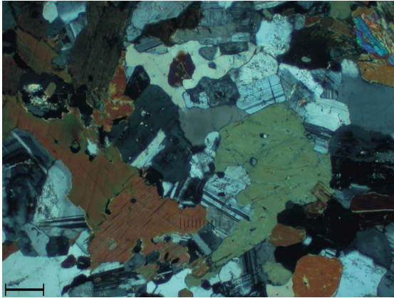
Fig. 71 - Gabbro appartenente alla tonalite del Monte Monoccola (TMX). Microfotografia a polarizzatori incrociati. Struttura eterogranulare ipidiomorfa con cristalli di orneblenda, biotite e plagioclasti labradoritici (scala di riferimento 350 \mu\text{m} ).
