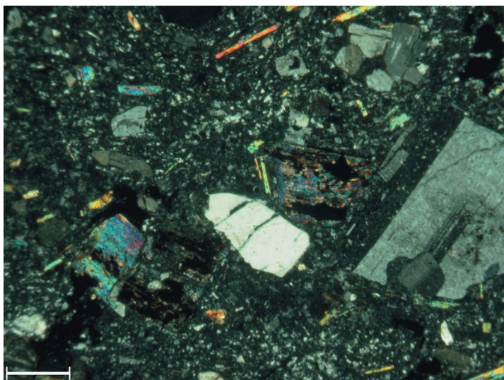
Fig. 43 - Formazione di Monte Macaone. Lava riodacitica. Associazione di plagioclasto, quarzo e biotiti in fondo microcristallino con orientamento fluidale. Microfoto a polarizzatori incrociati (scala di riferimento 675 \mu\text{m} ).
