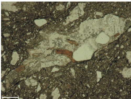
Fig. 39 - Litozona delle peliti con pomici. Visione generale, presenza di pomici inglobate da matrice pelitica microcristallina. Microfoto a polarizzatori paralleli (scala di riferimento 675 \mu\text{m} ).
