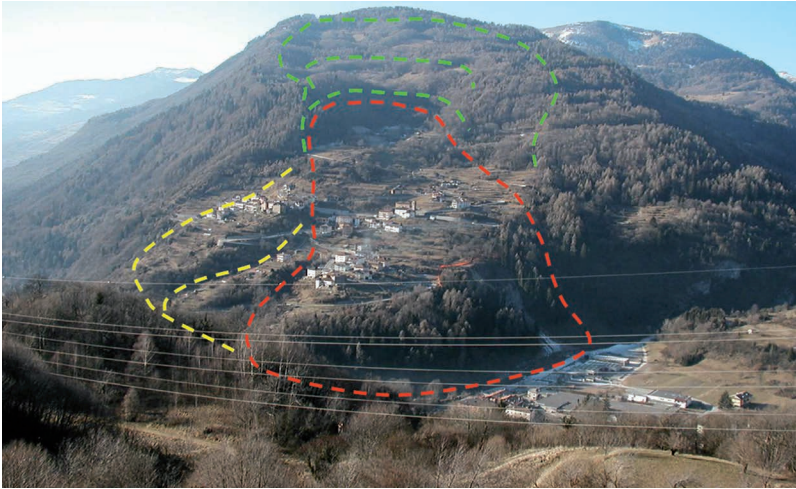
Fig. 98 - Panoramica del Monte Melino e dell'abitato di Prezzo, con evidenziata l'area di deformazione. Con tratteggio verde: antiche nicchie di distacco di frana; con tratteggio rosso e giallo: tre distinti corpi di accumulo di frana dalla forma convessa (foto ZAMBOTTO, 2002).
