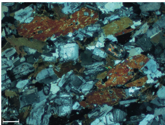
Fig. 66 - Gabbro-diorite del Complesso del Cornone di Blumone (GDA a ) . Microfotografia a polarizzatori incrociati, che mette in risalto la tessitura fortemente orientata con tendenza porfirica dei cristalli di orneblenda, associati a plagioclasti a nucleo bitownitico e bordo labradoritico (scala di riferimento 350 µm).
