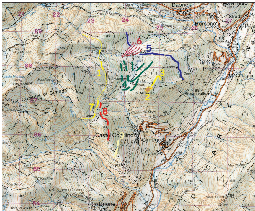
Fig. 79 - Mappa schematica dell'area di Buoniprati, con evidenziate le morene descritte nel testo; in giallo a tratteggio il limite LGM; numeri riferiti al testo.
