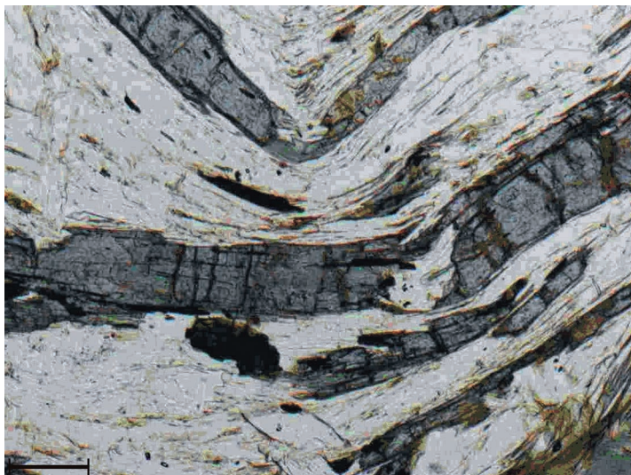
Fig. 26 - Cloritoide deformato e boudinato durante lo sviluppo di D_2 . Nel collo del boudin cresce clorite (polarizzatori paralleli, scala di riferimento 0,1 mm) (foto D. Zanoni).
