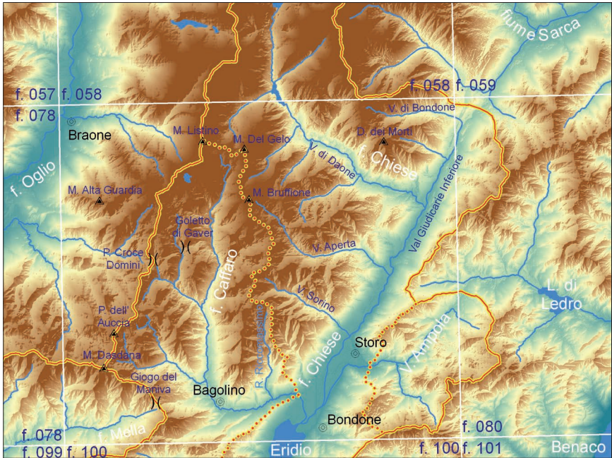
Fig. 11 - Inquadramento fisiografico dell'area del Foglio: assi di drenaggio principali e relativi spartiacque: in puntinato gli spartiacque di alcuni sottobacini. Elaborazione grafica S. Racchetti.
