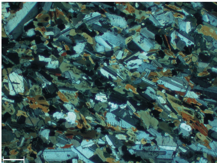
Fig. 64 - Filone lamprofirico picrobasaltico (fu). Microfotografia a polarizzatori incrociati. Struttura eterogranulare ipidiomorfa con elevata concentrazione di orneblenda e biotite associati a plagioclasio bitownitico (scala di riferimento 350 \mu\text{m} ).
