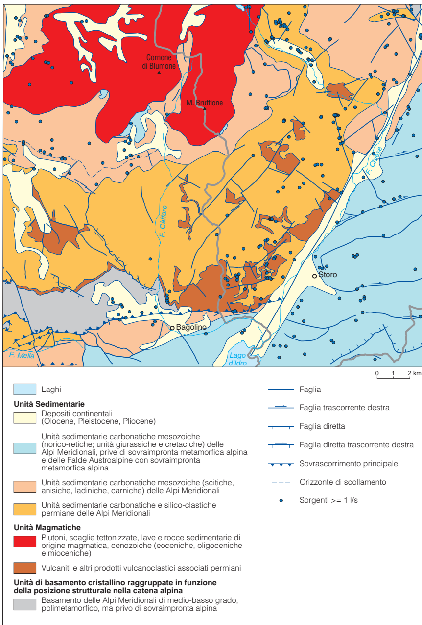
Fig. 105 - Principali sorgenti nel Foglio 079-Bagolino.
