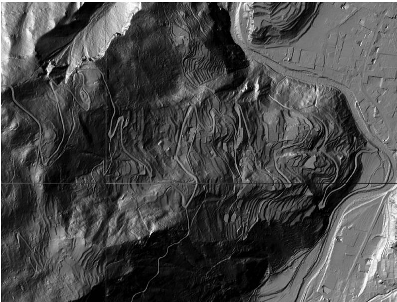
Fig. 99 - Estratto planimetrico del modello digitale del terreno con rilievo LIDAR, in cui si può osservare la frana di Prezzo (ZAMBOTTO, 2002).
