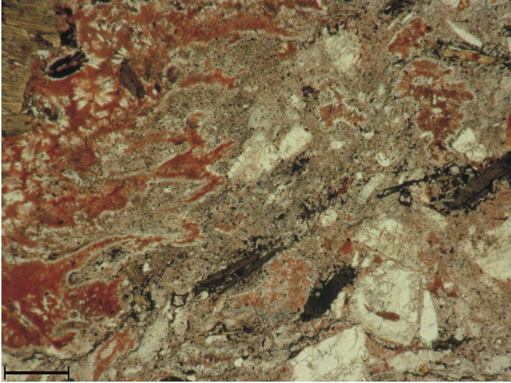
Fig. 51 - Vulcanite di Auccia - Litozona superiore. Particolare di fiamme interdigitate con il fondo ossidato. Microfoto a polarizzatori paralleli (scala di riferimento 250 \mu\text{m} ).
