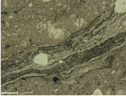
Fig. 33 - Fiamme pomicee rinaldate orientate lungo la direzione del flusso piroclastico. Microfoto a polarizzatori paralleli (scala di riferimento 125 \mu m).
