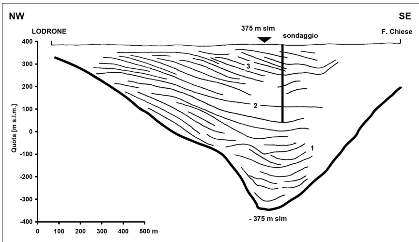
Fig. 23 - Interpretazione geologica del profilo sismico di Lodrone di Storo con l'ubicazione del sondaggio profondo (modificato da FELBER et alii , 2000).
