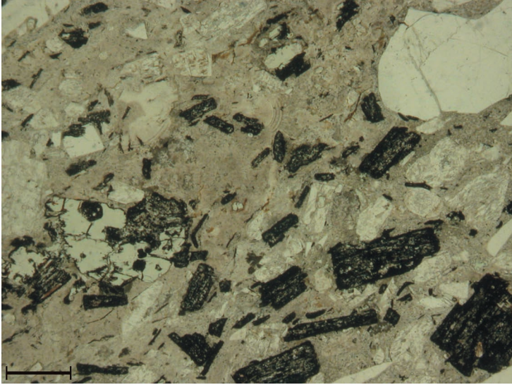
Fig. 48 - Vulcanite di Auccia - Litozona inferiore e intermedia. Ignimbrite con cristalli orientati di biotite, pirosseni, quarzo, plagioclasti. Microfoto a polarizzatori paralleli (scala di riferimento 675 \mu\text{m} ).
