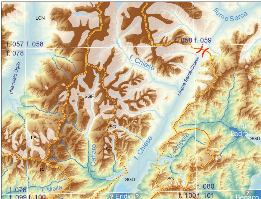
Fig. 17 - Schema dell'area del Foglio e delle aree limitrofe; in evidenza, l'estensione dei ghiacciai durante l'LGM, ricavabile dai sedimenti conservati e dalle geometrie ipotizzabili in base a essi. Spartiacque come in Fig. 11; in rosso, la sella di Bondo che mette in comunicazione il bacino del Sarca con quello del Chiese (dati desunti dai rispettivi Fogli pubblicati; elaborazione grafica F. Torri, S. Rachetti).
