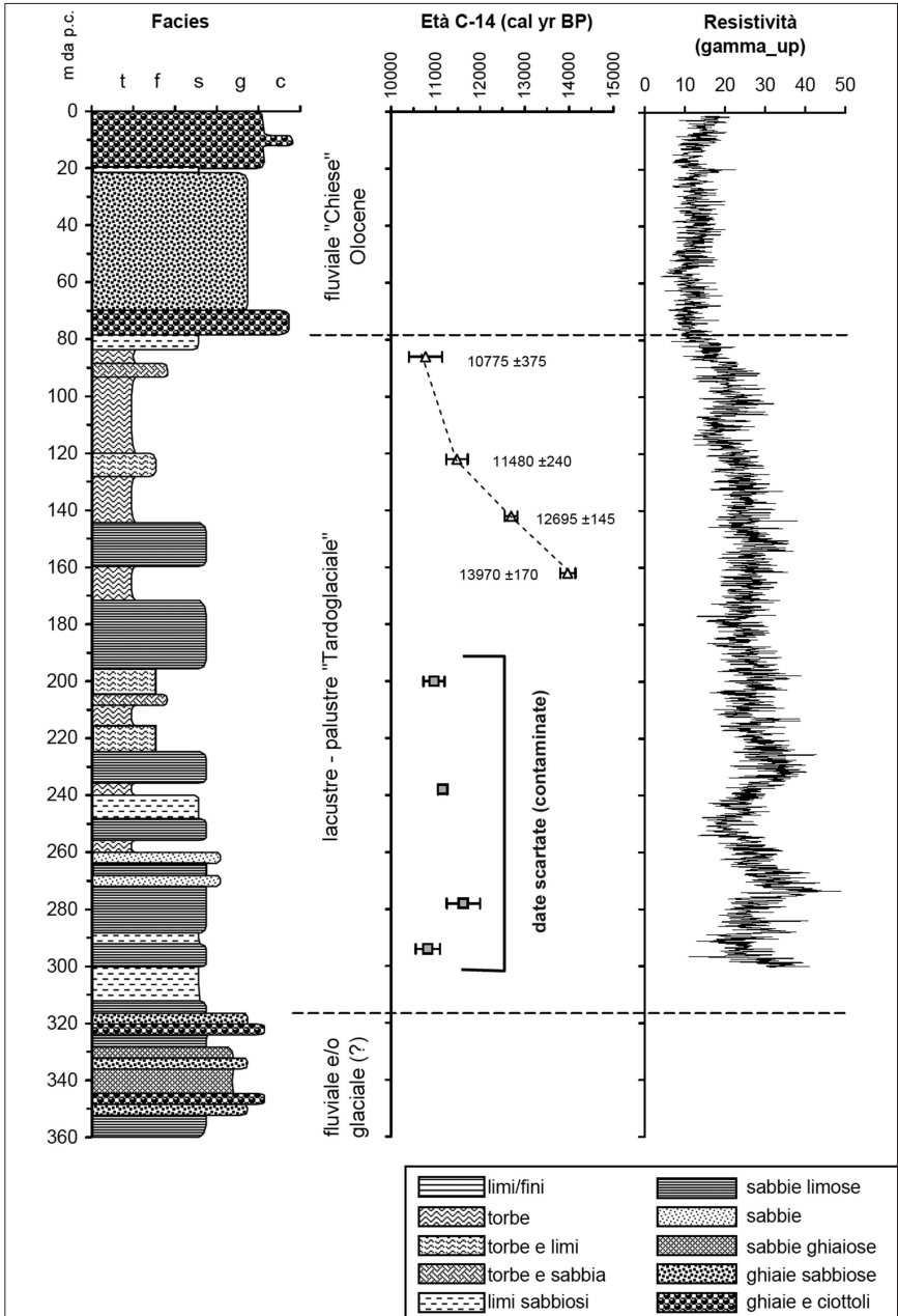
Fig. 24 - Stratigrafia, datazioni ^{14}\text{C} e log gamma-gamma del sondaggio Lodrone di Storo.
