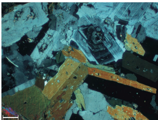
Fig. 70 - Diorite appartenente alla tonalite del Monte Monoccola (TMX). La microfotografia a polarizzatori incrociati mette in evidenza la struttura fanero-cristallina ipidiomorfa della roccia, ricca di biotite con orneblenda, plagioclasio labradoritico, quarzo e scarso feldspato alcalino (scala di riferimento 350 \mu m).
