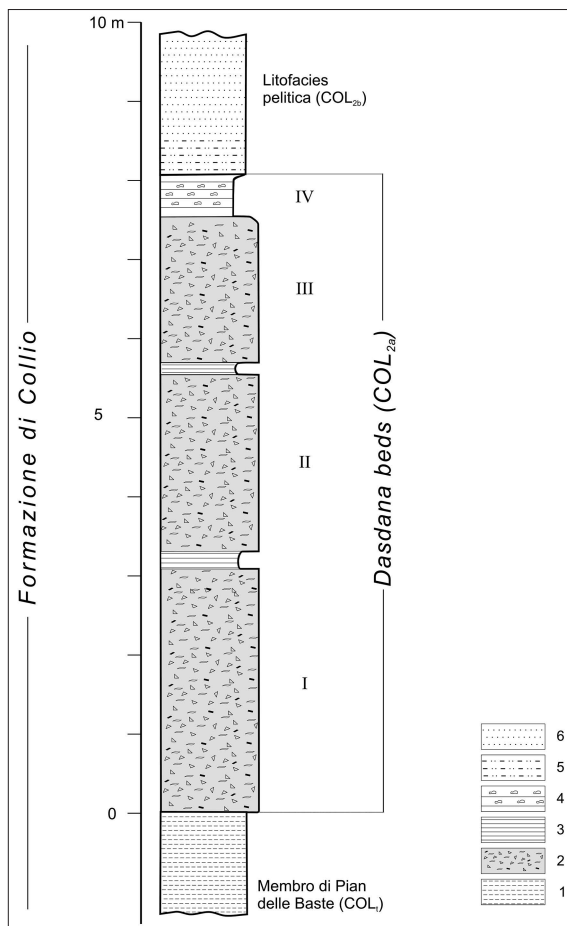
Fig. 35 - Colonna stratigrafica dei Dasdana beds, litofacies piroclastica del Membro di Val Dorizzo della Formazione di Collio (COL 2a ). Affioramento di Monte Dasdana, lungo la statale Maniva - Croce Domini. 1 - argilliti. 2 - ignimbrite. 3 - tufo. 4 - epiclastiti con livelletti di pomici. 5 - siltite. 6 - arenite. Modificato da Riguzzi (1996).
