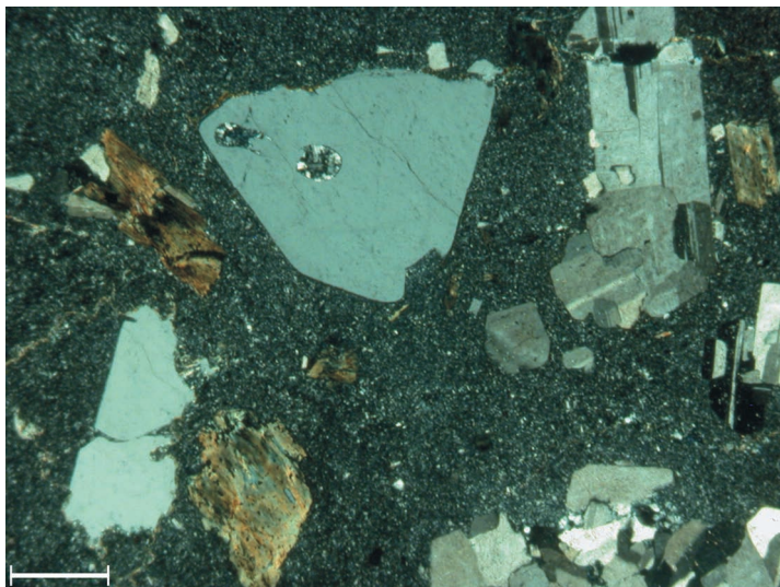
Fig. 42 - Formazione di Monte Macaone. Lava dacitica. Struttura porfirica con fenocristalli di quarzo, plagioclasti, biotite in fondo microgranulare cristallino. Microfoto a polarizzatori incrociati (scala di riferimento 125 \mu\text{m} ).
