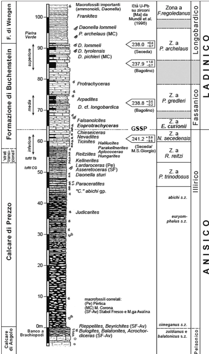
Fig. 107 - Colonna stratigrafica sintetica del Triassico medio esposta lungo l'alveo del Fiume Căffaro presso Romantera (Bagolino). La sigla GSSP indica il livello stratigrafico del "chiodo d'oro" della base del piano Ladinico (modificata da BRACK et alii, 2005). La denominazione delle sottozone (s.z.) per l'Anisico è da MONNET et alii (2008).
