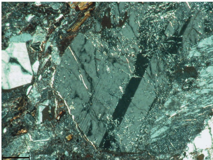
Fig. 53 - Vulcanite di Auccia - Litozona superiore. Particolare di cristallo di plagioclasio albitizzato. Microfoto a polarizzatori incrociati (scala di riferimento 250 \mu m).
