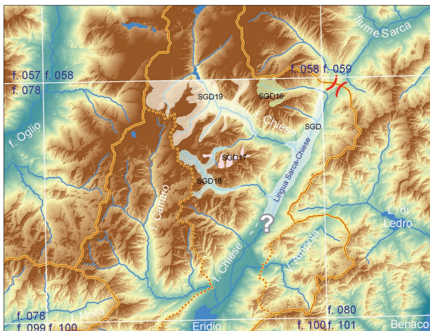
Fig. 20 - Sintema del Garda e suoi subsistemi durante le fasi di ritiro. Lo sgonfiamento della lingua Sarca-Chiese isola i ghiacciai delle valli laterali (Daone, Bondone), mentre i ghiacciai locali della Valle del Ribor e di Valle Aperta già separati si annidano alla testata delle rispettive valli (elaborazione grafica S. Rachetti).
