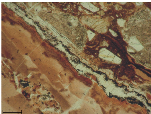
Fig. 58 - Ciottolo di selce nel conglomerato del Verrucano Lombardo a tetto della litozona superiore della vulcanite di Auccia a Punta dell'Auccia. Tali selci di origine idrotermale sono abbondanti negli ultimi episodi vulcanici della litozona superiore della vulcanite di Auccia. Microfoto a polarizzatori paralleli (scala di riferimento 675 \mu\text{m} ).
