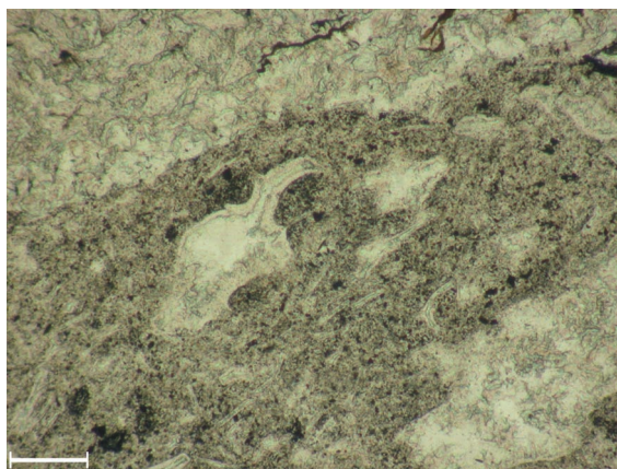
Fig. 32 - Shard vetrosi incurvati nella pasta di fondo di una fiamma. Microfoto a polarizzatori paralleli (scala di riferimento 125 µm).
