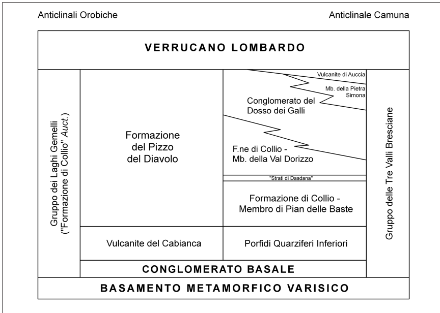
Fig. 29 - Schema della successione vulcano-sedimentaria affiorante nel settore delle anticlinali orobiche e camuna (Comitato d'area per le Alpi centrali, orientali ed occidentali, 2005).
