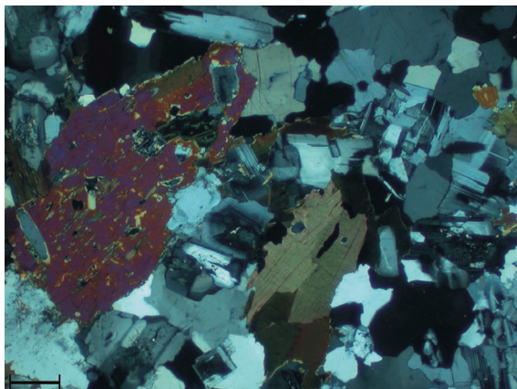
Fig. 67 - Tonalite del Monte Alta Guardia (TMG). Microfotografia a polarizzatori incrociati. Struttura granulare ipidiomorfa con abbondanti plagioclasti labradoritico-andesinici associati a biotite, orneblenda, quarzo e K-feldspato interstiziale (scala di riferimento 350 \mu\text{m} ).
