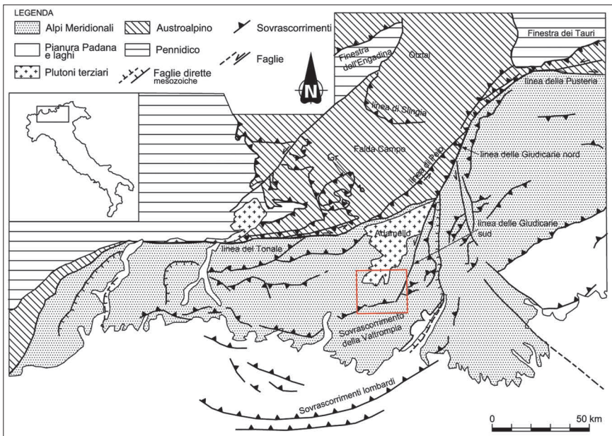
Fig. 7 - Schema tettonico delle Alpi Centrali e delle Alpi Meridionali (Sudalpino). La cornice indica la posizione del Foglio 079-Bagolino. Le faglie mesozoiche sono tratte da BERTOTTI et alii (1993).
