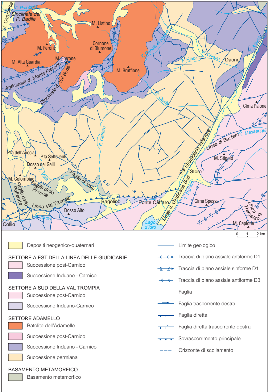
Fig. 92 - Schema tettonico del Foglio 079-Bagolino.
