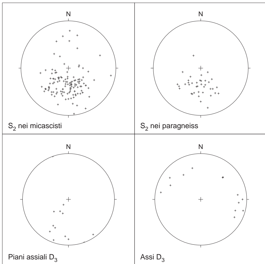
Fig. 89 - Proiezioni stereografiche degli elementi del fabric del basamento metamorfico (Reticolo di Schmidt su emisfero inferiore).
