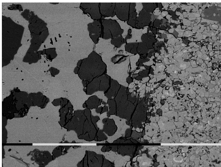
Fig. 76 - Breccia del Pissalat (BPA). Microfotografia SEM, scala di riferimento 0,1 mm. Dettaglio della fascia a silicati con cristalli di forsterite in calcite (lato destro) e associazione di granuli di diopside, calcite e tremolite (lato sinistro).
