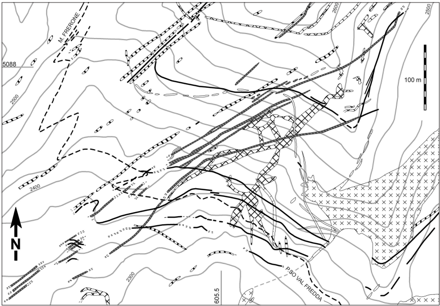
Fig. 9 - Rapporti di intrusione tra diverse generazioni di filoni sul versante meridionale del Monte Frerone. Per la legenda vedi Fig. 8 (da BRACK, 1981).
