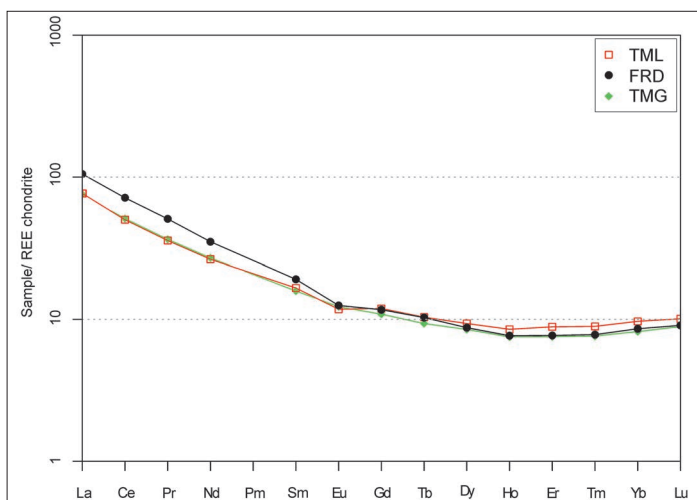
Fig. 74 - Pattern delle Terre Rare delle rocce intrusive del plutone Re di Castello nel Foglio 079-Bagolino. I valori sono normalizzati alla Chondrite C1 (SUN & Mc DONOUGH, 1989).
