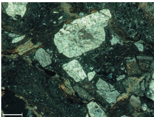
Fig. 38 - Membro di Val Dorizzo - Litofacies piroclastica. Plagioclasti idiomorfi associati a biotiti deformate. Microfoto a polarizzatori incrociati (scala di riferimento 400 \mu\text{m} ).
