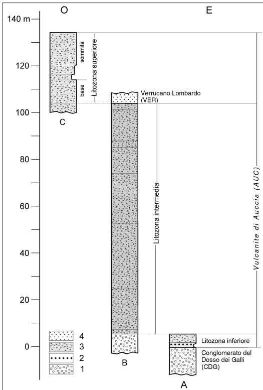
Fig. 47 - Colonne stratigrafiche della vulcanite di Auccia (AUC). A- Serie di Dosso dei Galli. B- Serie di Punta dell'Auccia (E e S). C- Serie di Punta dell'Auccia (N). 1 - conglomerato. 2 - tufo grossolano. 3 - ignimbrite. 4 - arenaria. Modificate da CASSINIS (1968c) e da PEROTTI (1995).
