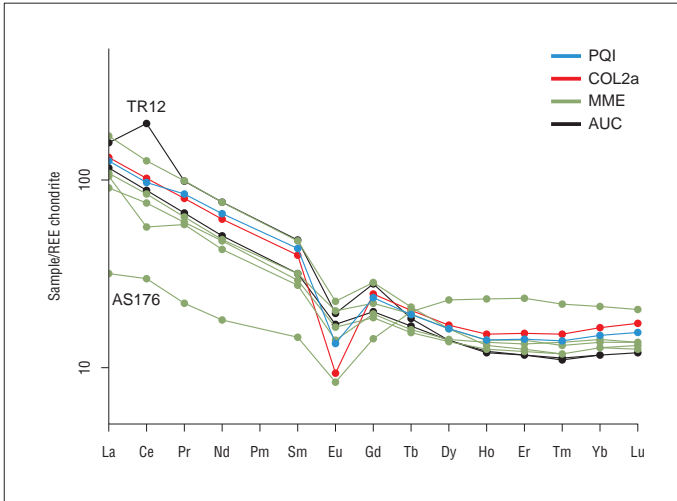
Fig. 56 - Pattern delle Terre Rare delle vulcaniti permiane del Foglio 079-Bagolino. I valori sono normalizzati alla Condrite (C1), SUN & Mc DONOUGH (1989).
