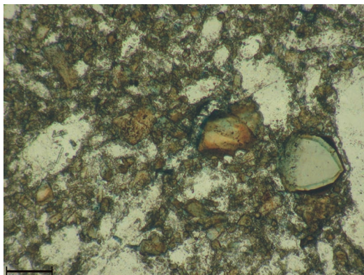
Fig. 57 - Conglomerato del Verrucano Lombardo (VER) a tetto della litozona superiore della vulcanite di Auccia a Punta dell'Auccia. Ciottoli di colore verde scuro e nerastro costituiti da quarzo e tormalina. Ciottoli analoghi si riscontrano anche nel Conglomerato della Val Daone (VER1). Microfoto a polarizzatori paralleli (scala di riferimento 125 \mu\text{m} ).
