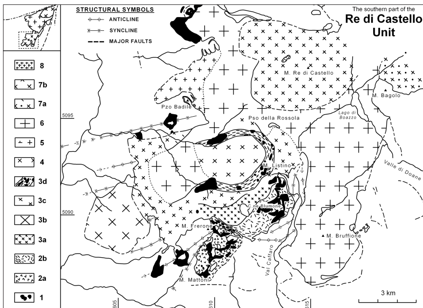
Fig. 8 - Schema della struttura interna della "superunità" del Monte Re di Castello e delle strutture pre- e sin-intrusive. Unità intrusive in ordine di intrusione, dal più antico: 1. gabbri; 2a. leucotonaliti-trondhjemititi della Val Fredda; 2b. complesso del Blumone; 3a. tonaliti del Lago della Vacca; 3b. tonalite del Monte Alta Guardia; 3c. tonaliti a grana fine; 3d. struttura anulare del Listino; 4. tonalite del Listino; 5. granodiorite del Badile; 6. granodioriti e leucotonaliti del Bruffione - Boazzo - Lago d'Arno; 7a. tonalite della Val Bona; 7b. tonalite del Monte Re di Castello; 8. trondhjemititi e graniti. (da BRACK, 1985).
