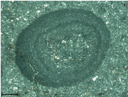
Fig. 34 - Cineriti con lapilli di accrezione con morfologia tondeggianti e zonazione concentrica a grana variabile. Microfoto a polarizzatori incrociati (scala di riferimento 675 \mu m).
