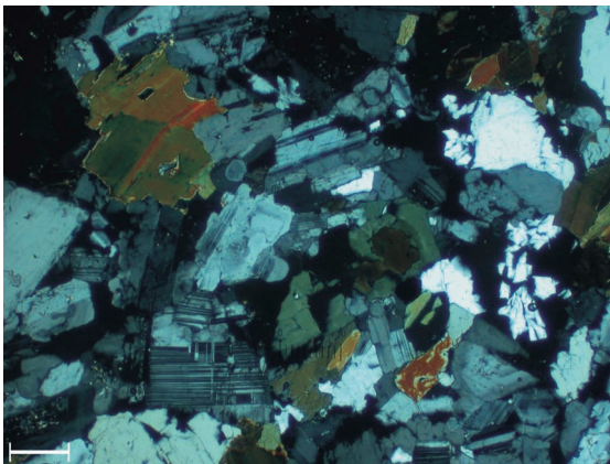
Fig. 69 - Tonalite del Lago della Vacca (LGV). Microfotografia a polarizzatori incrociati. Struttura granulare ipidiomorfa con abbondanti plagioclasti labradoritico-andesinici associati a biotite, orneblenda e quarzo (scala di riferimento 350 µm).
