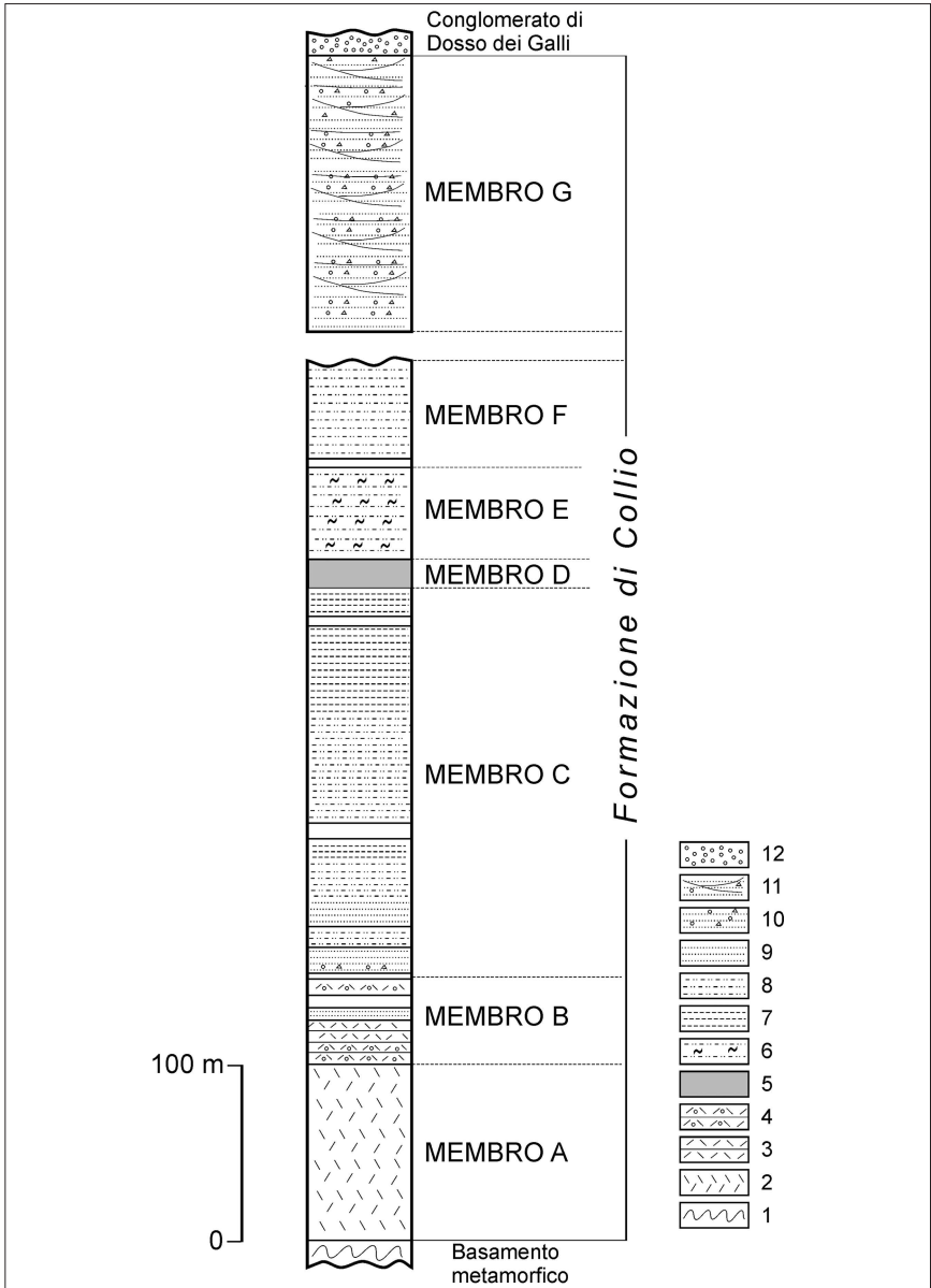
Fig. 3 - Colonna stratigrafica della sezione tipo della Formazione di Collio, modificata da CASSINI (1966a). 1 - Metamorfico, 2 - Ignimbrite, 3 - Tufo, 4 - Tufo a lapilli, 5 - Lava, 6 - Siltite con pomici, 7 - Argillite, 8 - Siltite, 9 - Arenaria, 10 - Arenaria con breccia e puddinga, 11 - Conglomerato poligenico e arenaria, 12 - Conglomerato.
