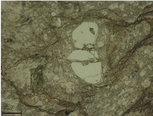
Fig. 37 - Membro di Val Dorizzo - Litofacies piroclastica. Quarzo fratturato e dislocato. Microfoto a polarizzatori paralleli (scala di riferimento 400 \mu\text{m} ).
