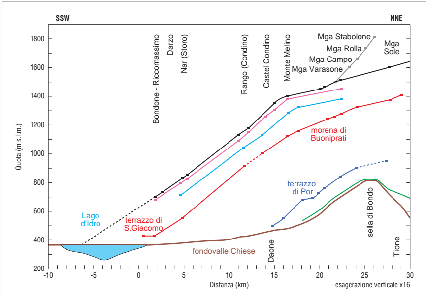
Fig. 19 - Profilo lungo l'asse giudicariense, tra il Lago d'Idro e Tione. La linea nera rappresenta il limite massimo LGM ricostruito in base ai depositi glaciali (Sintema del Garda). La linea grigia rappresenta la proiezione del limite LGM in Valle di Daone; quelle rosa e azzurra l'andamento del ghiacciaio durante le prime fasi di riavanzata glaciale a seguito dell'LGM. La linea rossa rappresenta l'andamento del ghiacciaio durante la riavanzata glaciale della fase di Buoniprati, quella blu l'andamento del ghiacciaio trasfidente dalla Val Rendena al momento della separazione della lingua glaciale proveniente dalla Valle di Daone (fase di Por). La linea verde rappresenta l'andamento dei depositi di contatto glaciale (versante Tione) e la piana torrentizia e di debris-flow (versante Daone) successiva alla disattivazione della sella di Bondo (fase di Tione, subsintema di Malè SGD 1 ).
