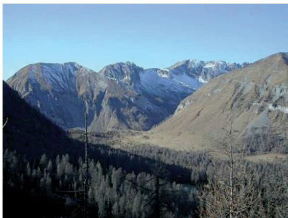
Fig. 84 - La sella di Bondolo (q. 1944 m) e la porzione alta della Valle di Malga Clevét con il Monte Remà (q. 2375) all'estrema destra. Alla base delle ampie falde detritiche del M. Remà si osserva la morena laterale sinistra e i depositi glaciali (SGD 17 ) relativi alla lingua transfluente dalla Val Aperta, della quale si vede sullo sfondo la cresta tra Cima Bondolo e il Monte Bruffione (foto A. Borsato).
